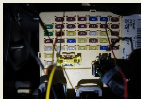
⑥ B+선을 정지등에 연결 * 정지등이 없을 경우, 시트히터조수석, 트렁크 순으로 퓨즈연결
