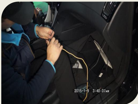
③ 전원선을 도구를 이용하여 조수석으로 이동
