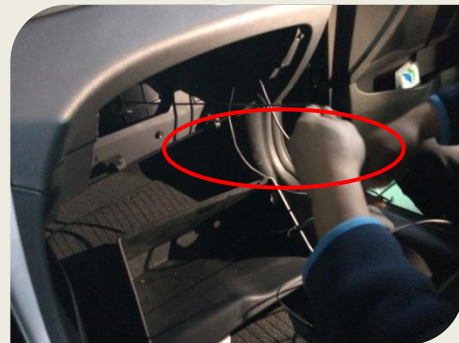
④ 전원선을 글로브박스 안으로 이동
